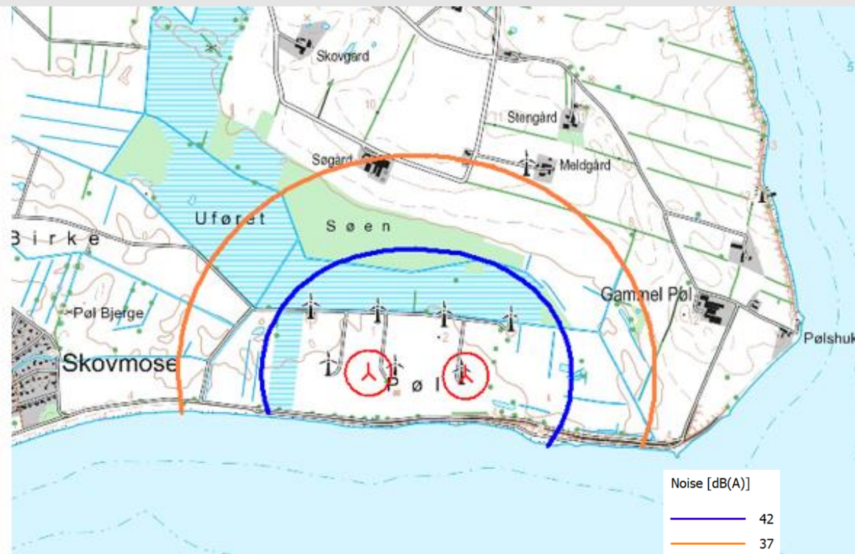
Støj Vindmøller (6 m/s) – 180 m høje møller
